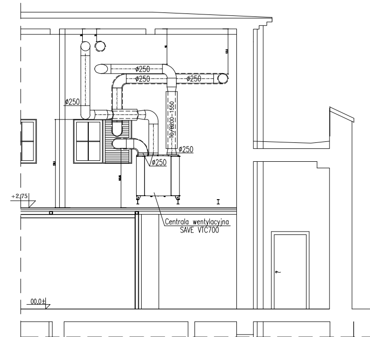
PRZEKRÓJ B-B
